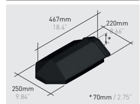
Q122*K | Angular hip / end ridge klinker
