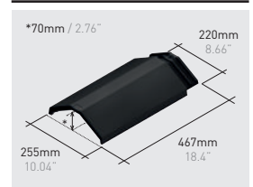
Q120*K | Angular ridge klinker
