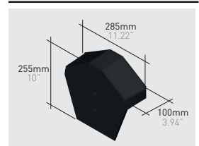
Q124*K | Angular end cap klinker
