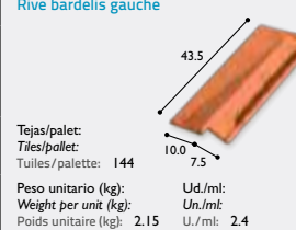
Remate lateral oblicuo izquierdo Left oblique lateral auction Rive bardelis gauche
