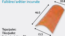
Caballette curvo Curved ridge Faîtière/arêtier incurvé
