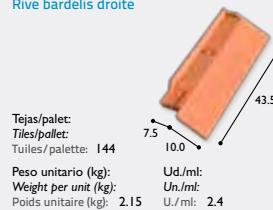
Remate lateral oblicuo derecho right oblique lateral auction Rive bardelis droite
