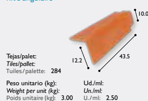
Remate angular Universal verge Rive angulaire
