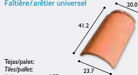
Caballette universal Universal ridge Faîtière/arêtier universel
